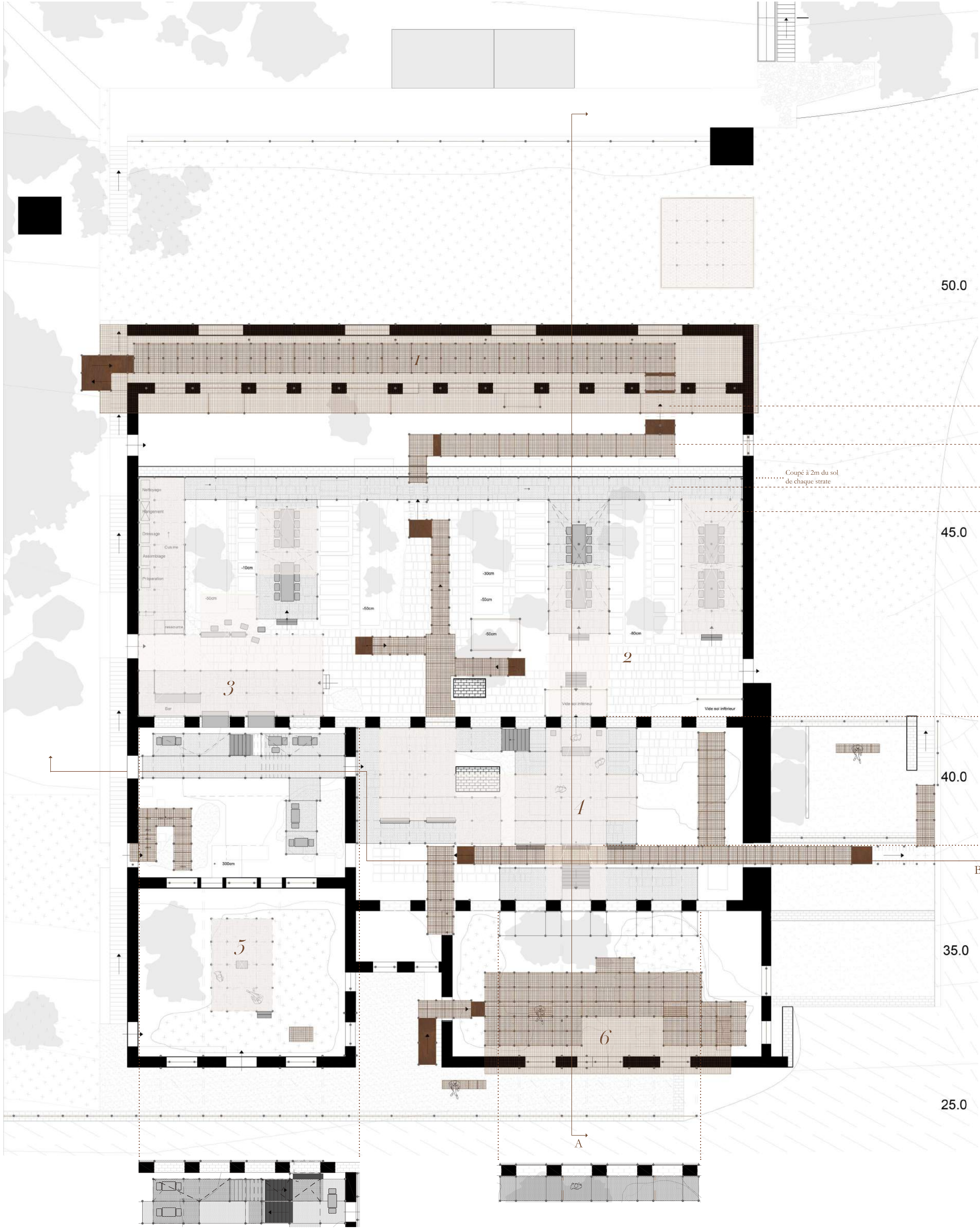
Plan de site 1:100 ème
