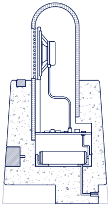
COUPE AA'
