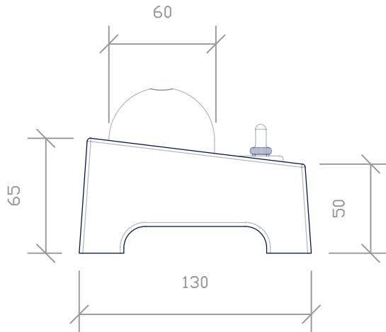
ÉLEVATION DE FACE
