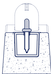
COUPE AA'
