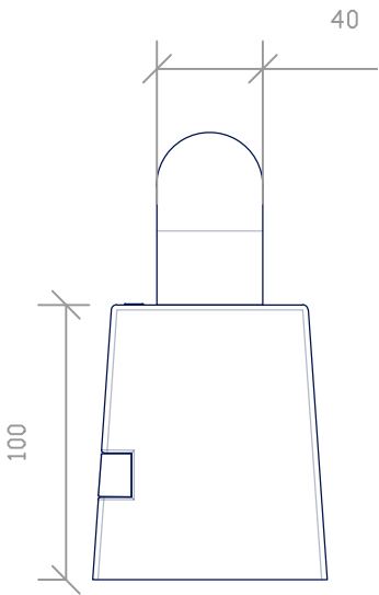
ÉLÉVATION DE CÔTÉ
