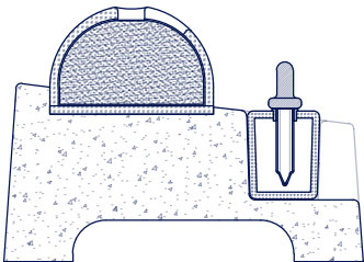
COUPE BB'
