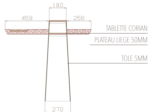
coupe BB' échelle 1/20
