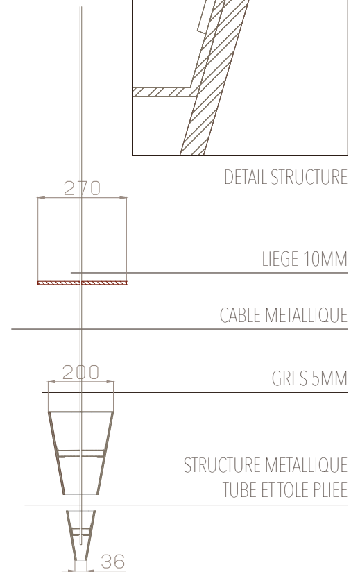
coupe BB'. échelle 1/16
