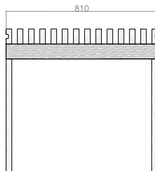
partie coulissante
