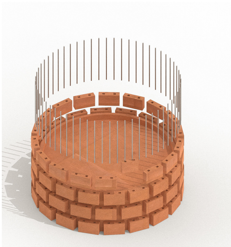
03-Assemblage briques et tiges métalique
