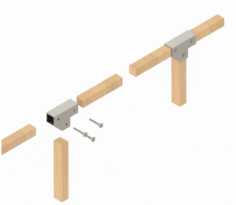
03-Assemblage Tasseaux pièces métallique
