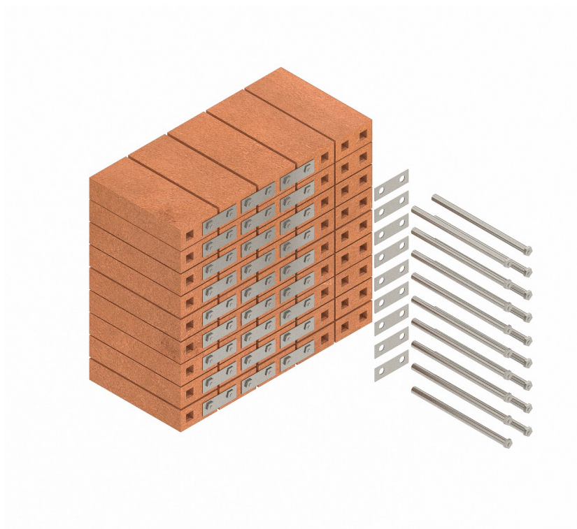
02-Assemblage des briques de la banquette
