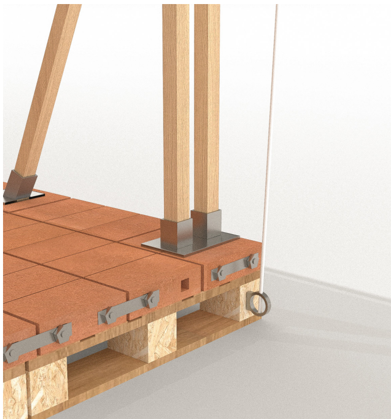
01-Assemblage de briques et palettes.
