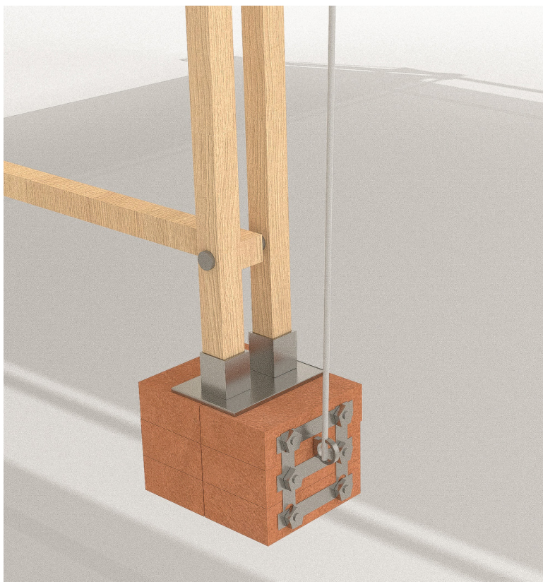
03-Plot de fixation pour tasseaux en brique et assemblage fils en tension et pièce métallique
